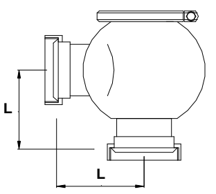
DIN MASCHIO DIN MALE
