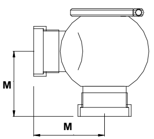
DIN FEMMINA DIN FEMALE
