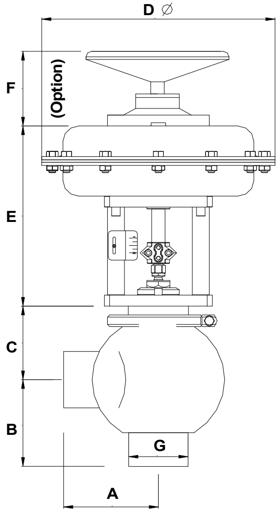
FLANGIA FLANGE
